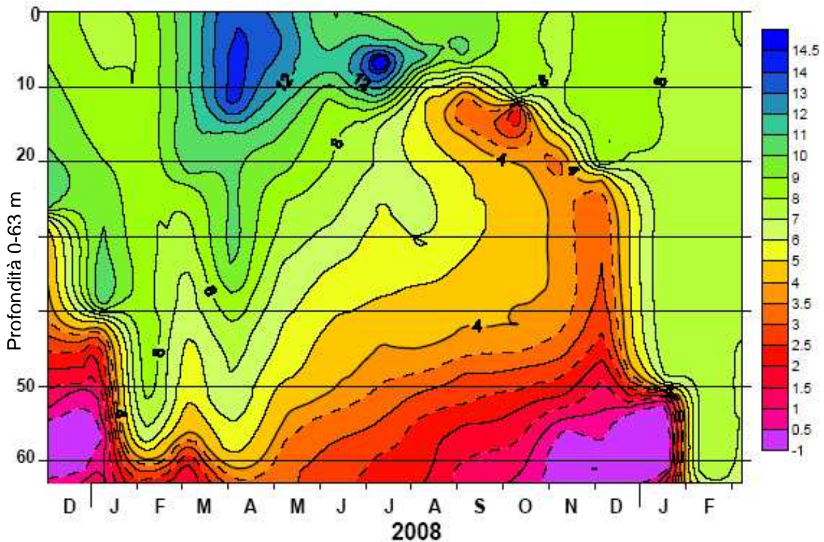
Figura 2: Grafico delle isoplete dell'ossigeno.
