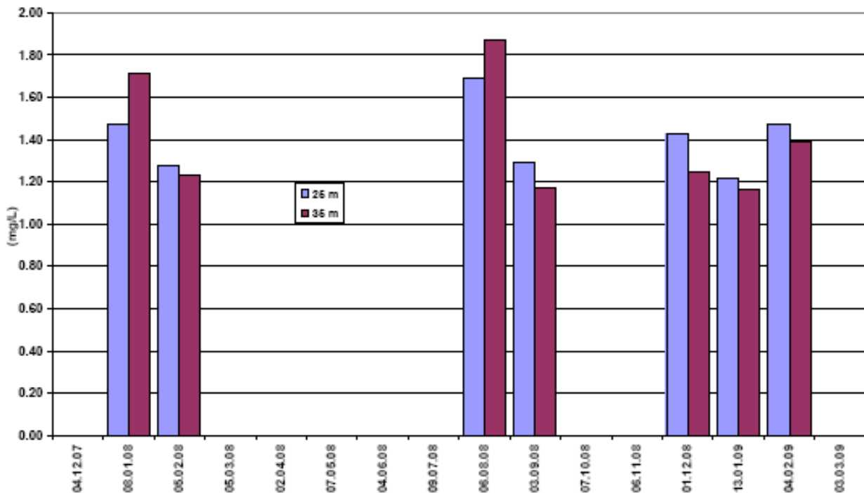
Figura 8: Carbonio organico disciolto a 25 e 35 m di profondità
