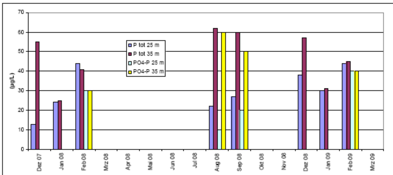
Figura 3: Concentrazioni di fosforo totale e fosfato-P a 25 e 35 m di profondità
