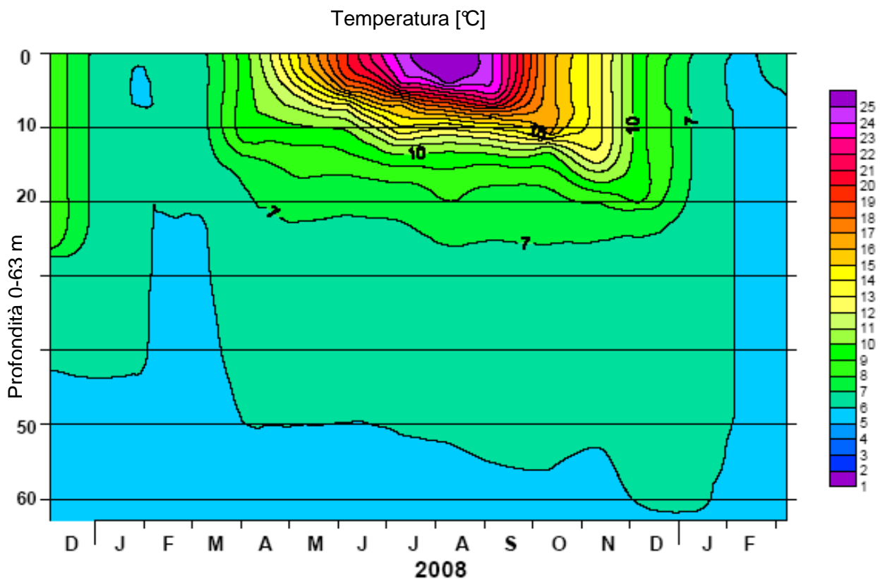
Figura 1: Grafico delle curve di temperatura
