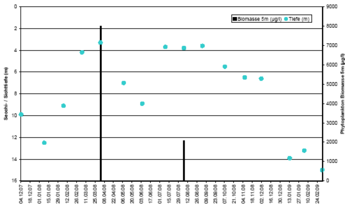
Figura 7: Trasparenza ("disco di Secchi") e biomassa del fitoplancton a 5 m di profondità
