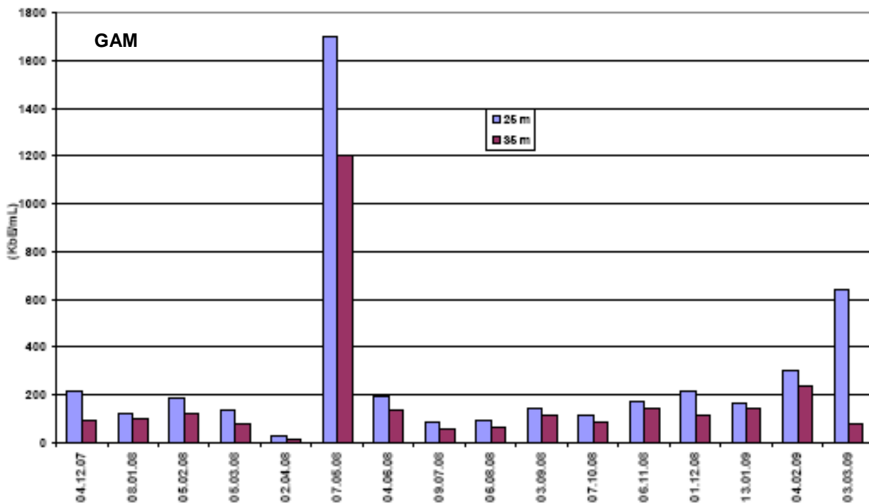
Figura 5: Germi aerobi mesofili a 25 e 35 m di profondità
