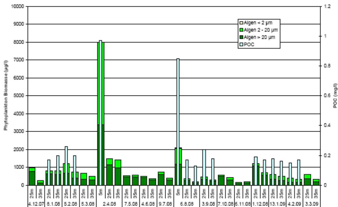
Figura 6: Biomassa del fitoplancton e carbonio organico particolato alle diverse profondità
